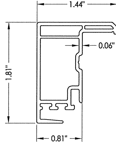
7 LOCK STILE
