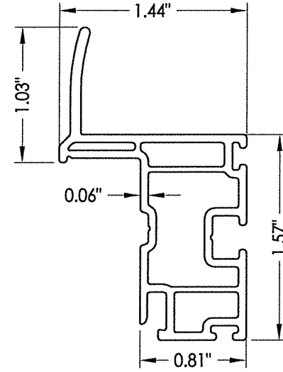
8 HANDLE STILE
